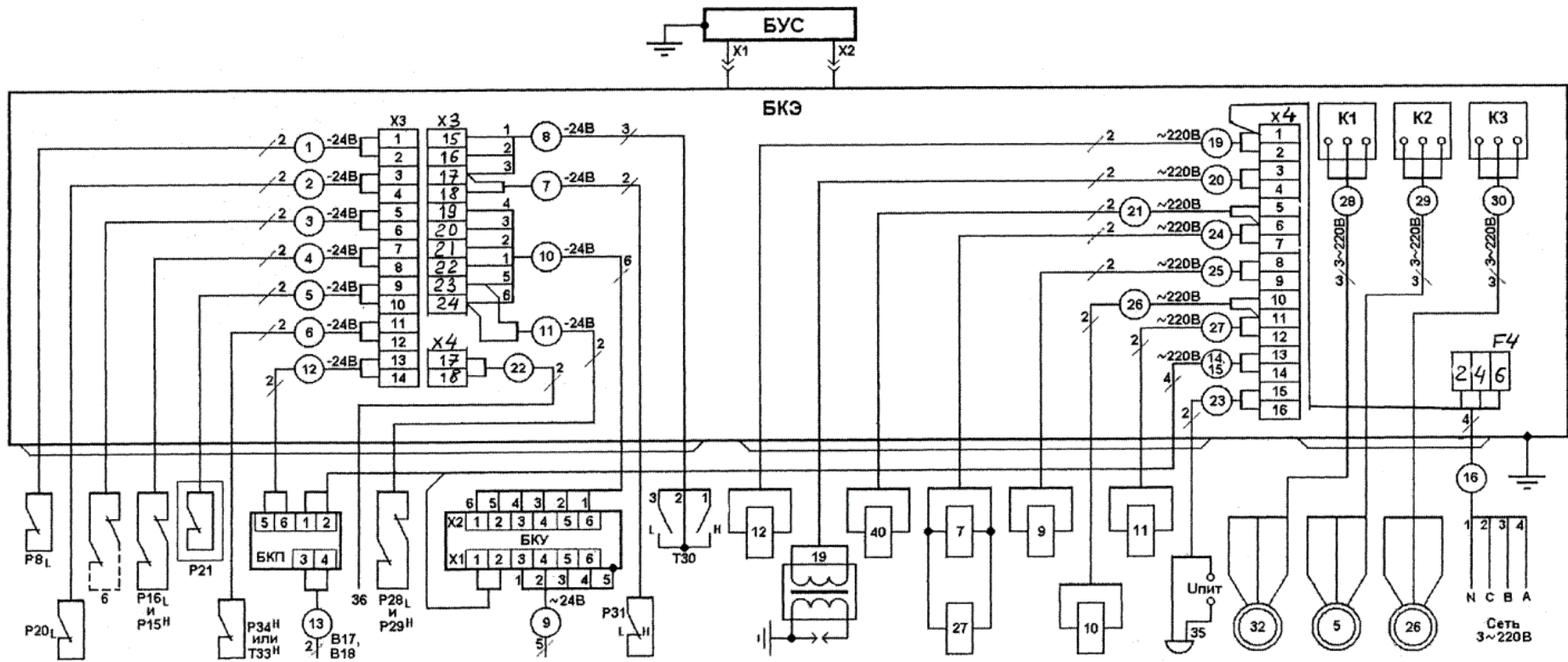
Схема подключений блока в одногорелочной тепловой установке
