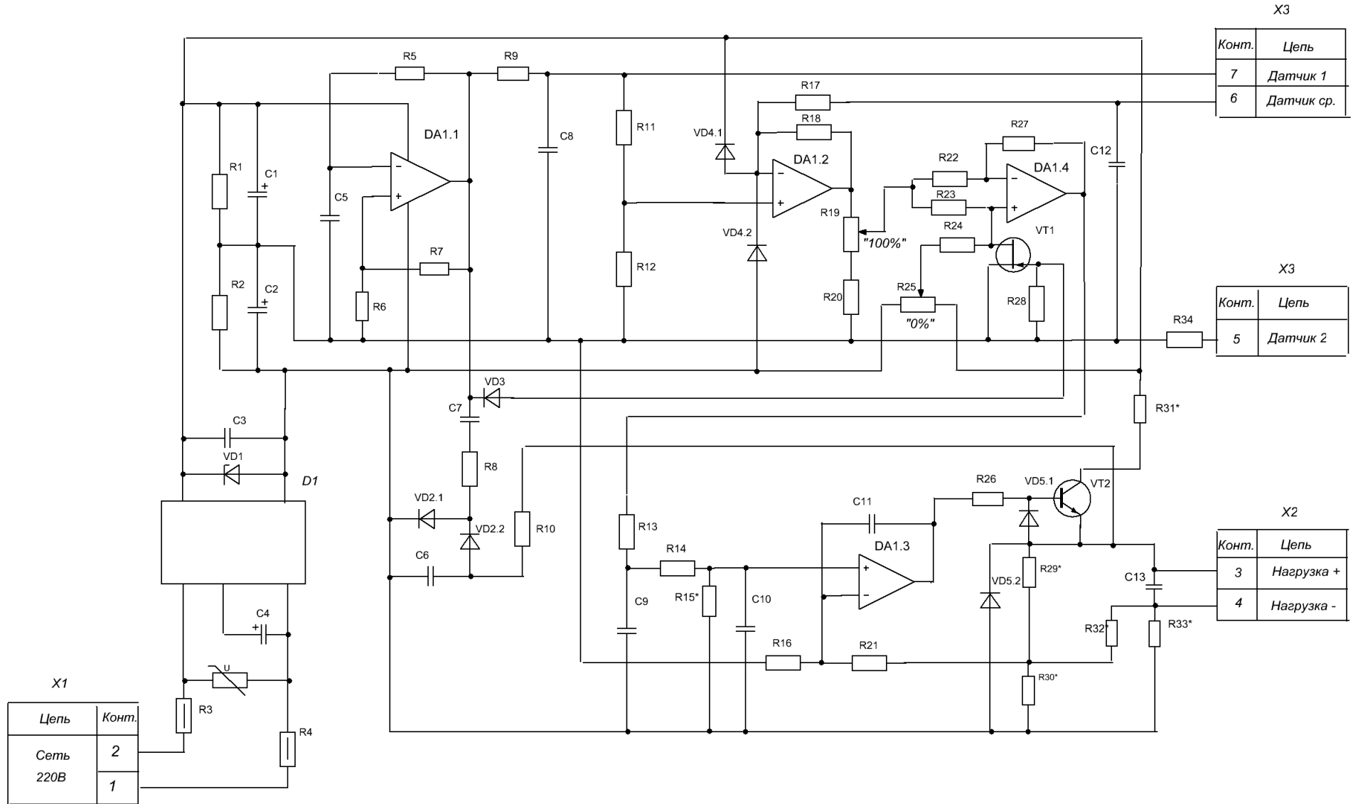
Схема электрическая принципиальная БУ-30М1И, БУ-30М1Р
